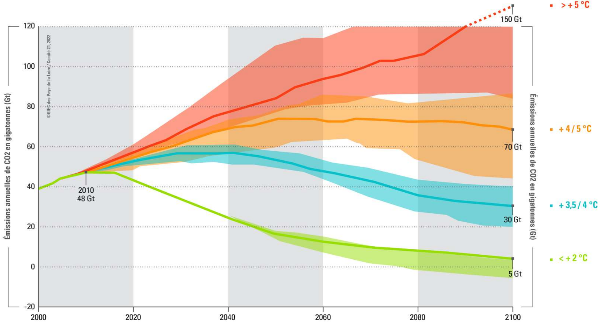
FIG. 6 • SCÉNARIOS D'ÉVOLUTION DES TEMPÉRATURES MONDIALES
