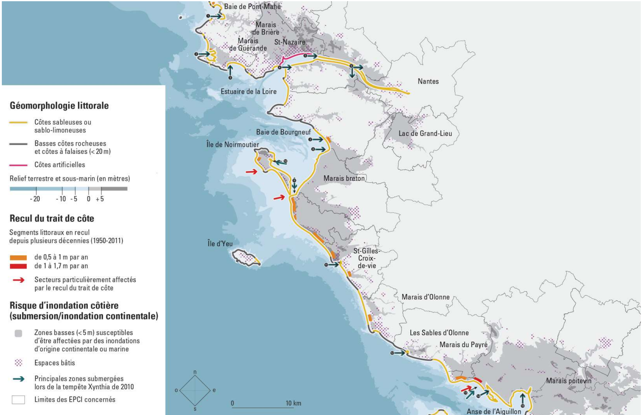
FIG. 23 • RISQUES DE SUBMERSION MARINE DANS LES PAYS DE LA LOIRE
